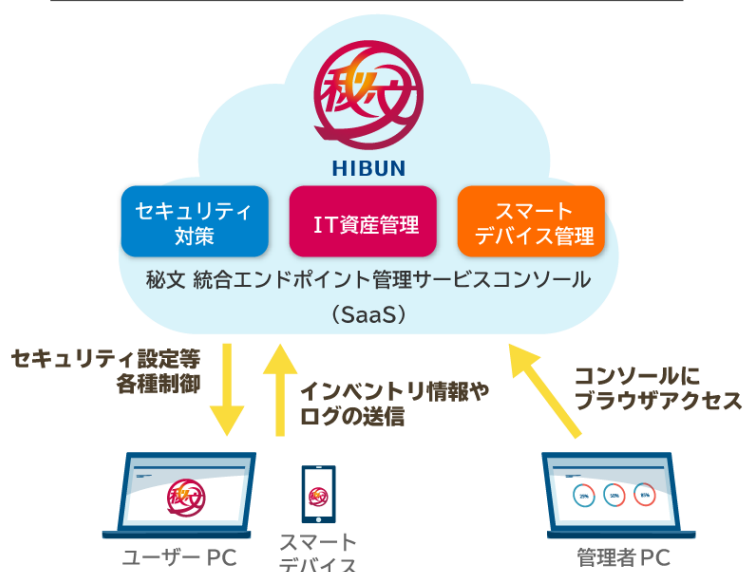
「秘文 統合エンドポイント管理サービス」システム構成図
