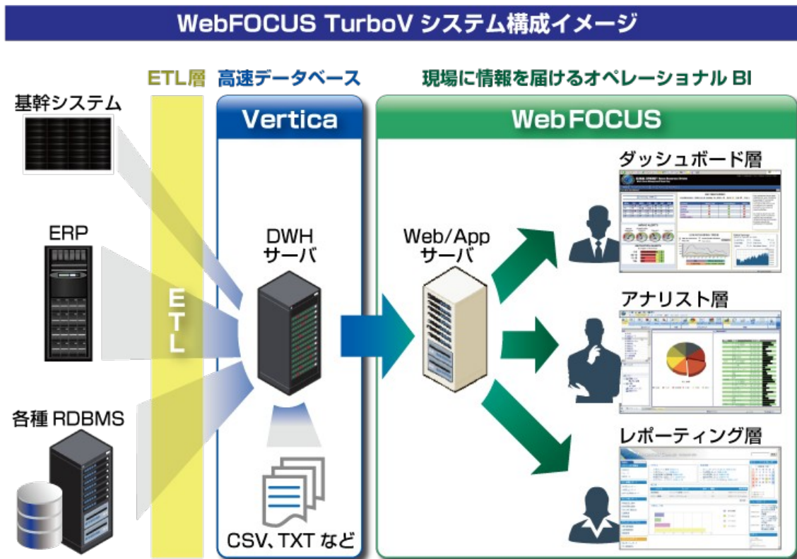
WebFOCUS TurboV システム構成図
